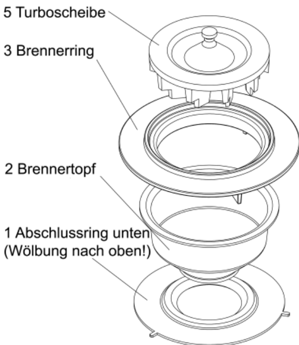
Abb. 20: Der Turbobrenner
