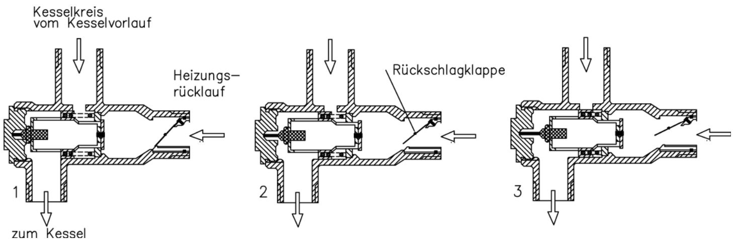
Abb. 15: Thermomix-Ventil Funktionsschema
