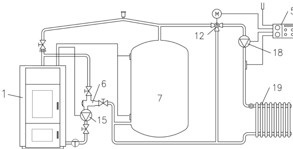
Abb. 16: Anlagenschema (Beispiel)
