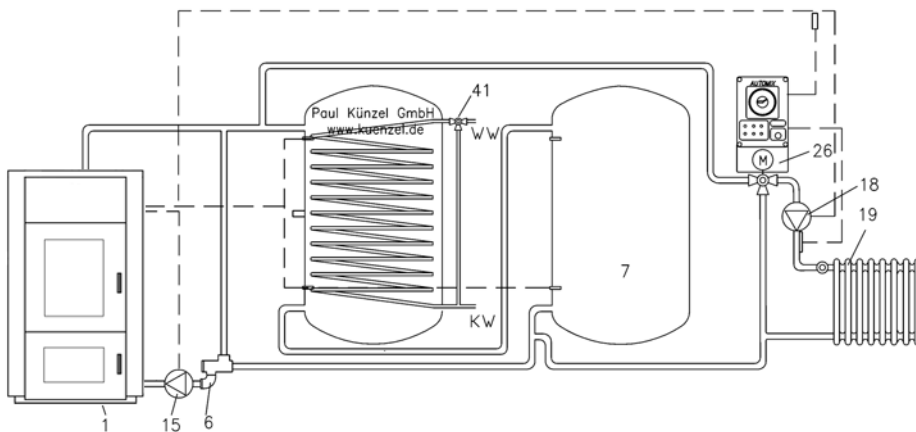
Abb. 41: Hydraulikschema für Systempaket A2
