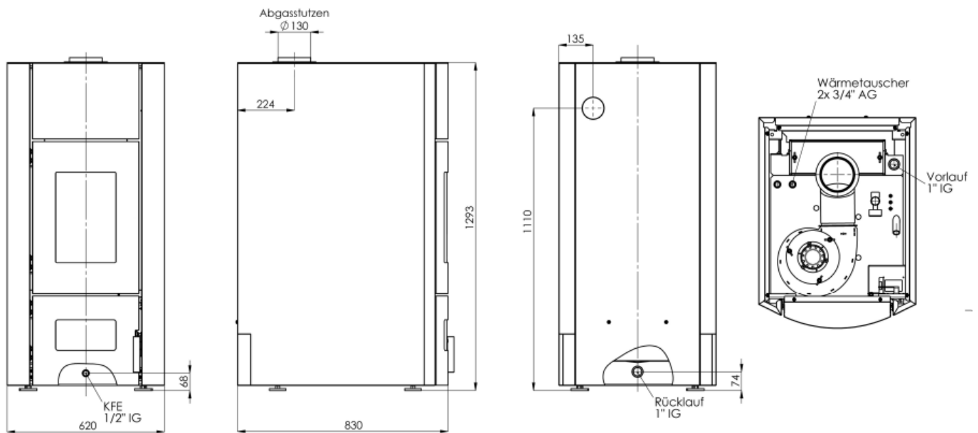
Abb. 40: Abmessungen HV-W / HV-H
