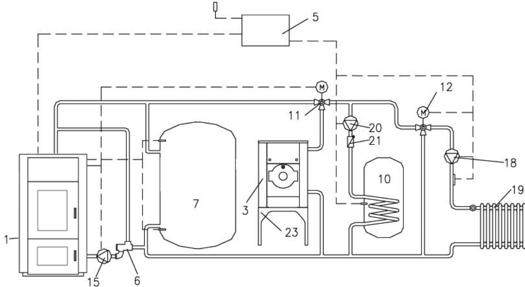
Abb. 42: Hydraulikschema für Systempaket F1
