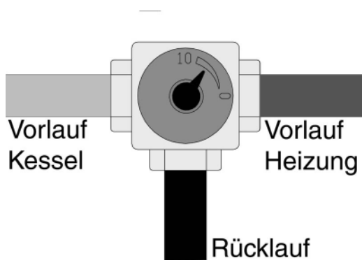
Abb. 7: Der Mischer in einer Zwischenstellung
