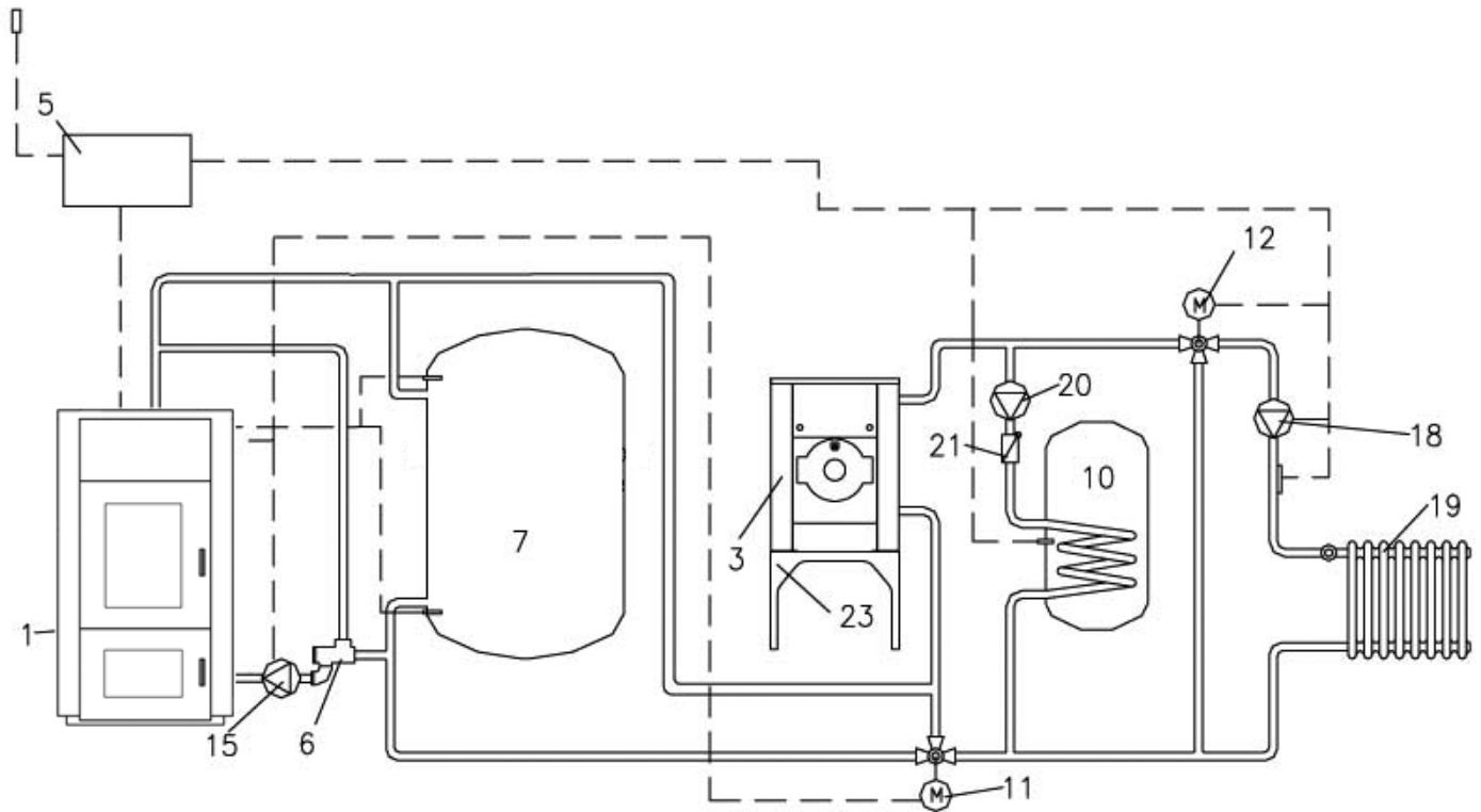
Abb. 44: Hydraulikschema nach Systempaket S11
