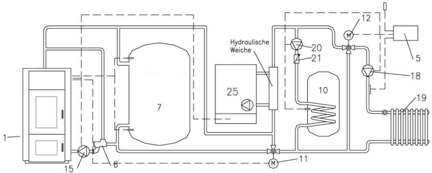
Abb. 45: Hydraulikschema nach Systempaket S13
