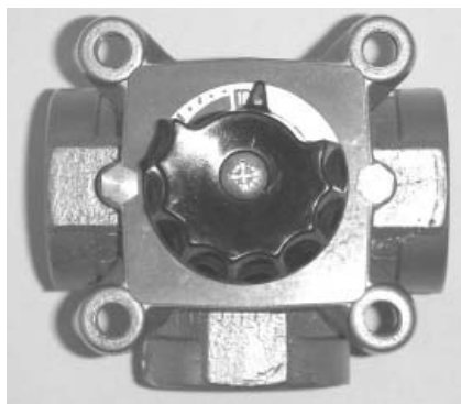
Abb. 8: Der KÜNZEL-Heizungsmischer
