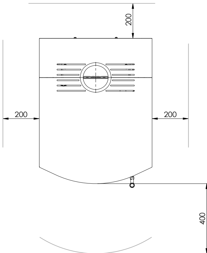
Abb. 1: Sicherheitsabstände im Aufstellraum in mm
