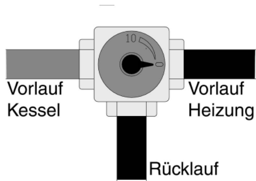
Abb. 6: Stellung „Durchgang Rücklauf“
