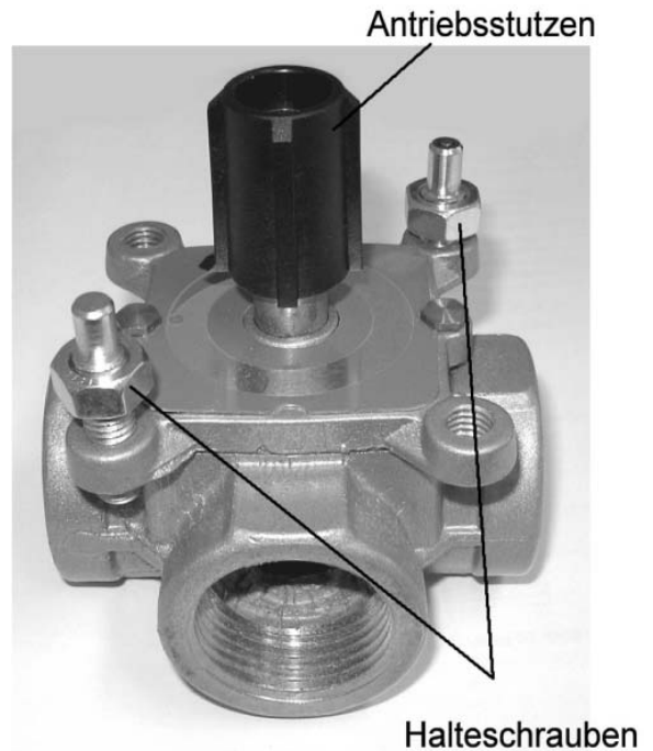
Abb. 13: Der Mischer
