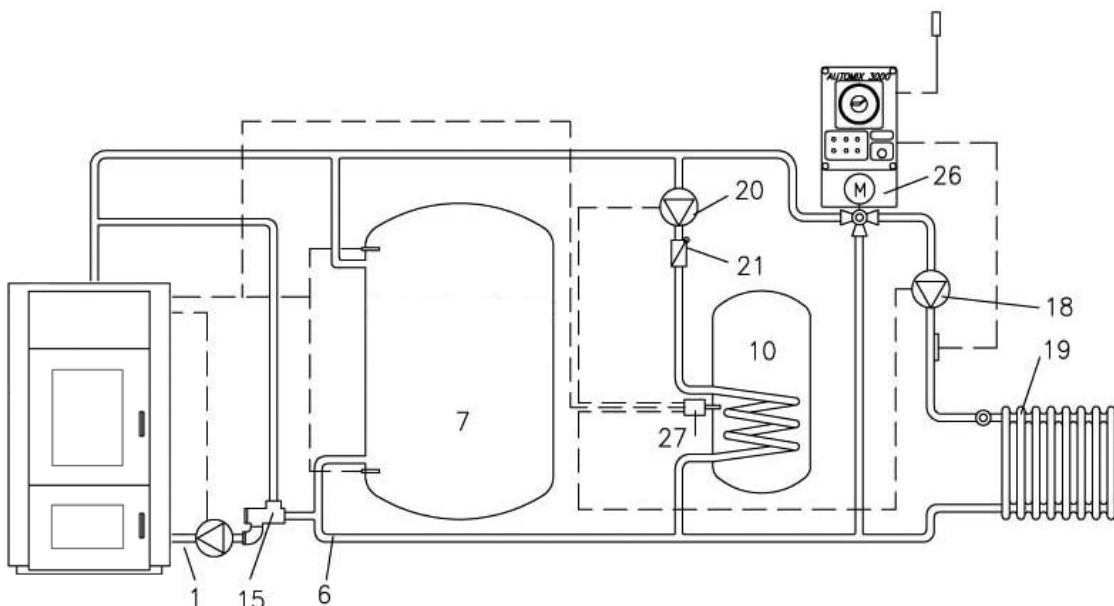
Abb. 43: Hydraulikschema nach Systempaket G1
