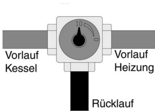
Abb. 5: Stellung „Durchgang Vorlauf“
