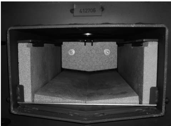
Abb. 29: Aschekasten hinten in der Brennkammer
