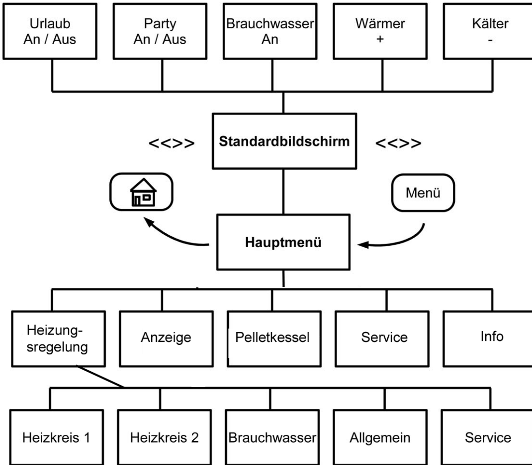
Abbildung 9: Der Menüaufbau
