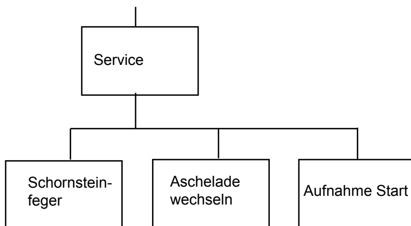
Abbildung 20: Untermenü Service
