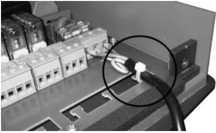
Abbildung 7: Zugentlastung
