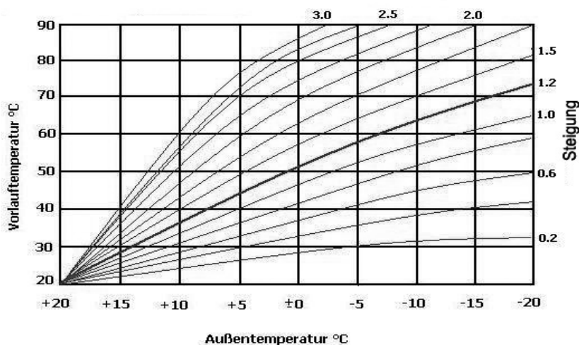
Abbildung 14: Heizkurve, Heizkennlinie
