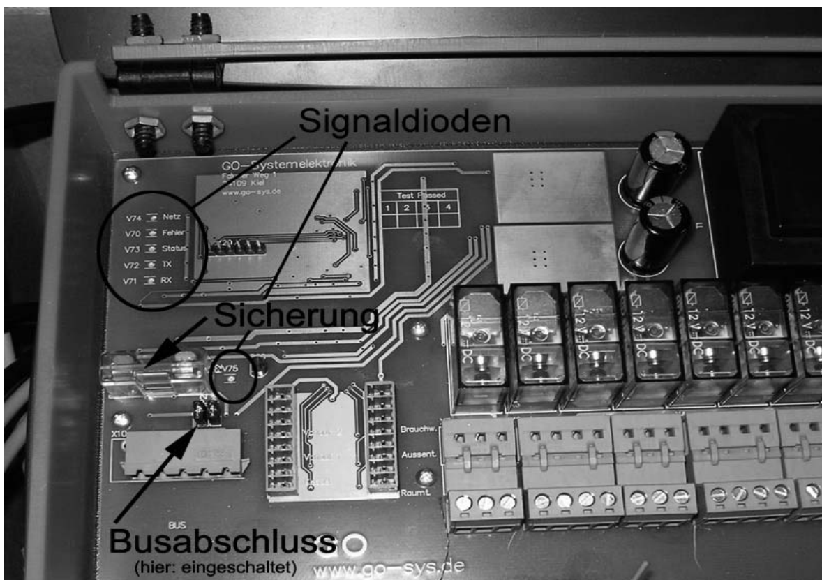
Abbildung 8: Die Platine der BD 600 A-PK
