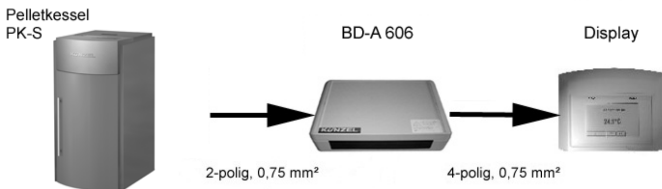
Abbildung 3: Verkabelung von PK-S, BD-A 606 und Touchscreen-Display
