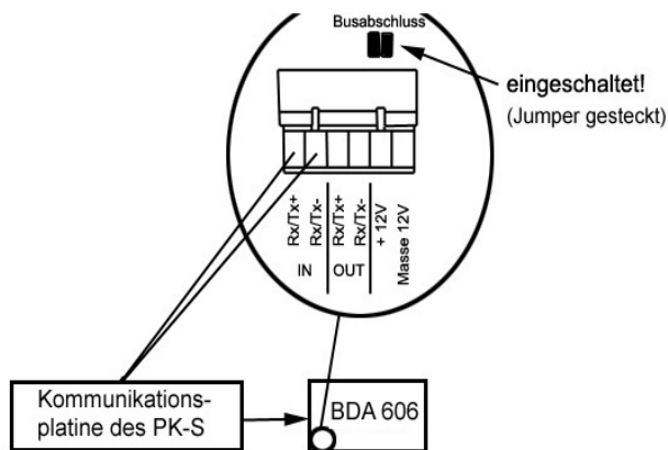
Abbildung 4: Kopplung Kommunikationsplatine und BD-A 606
