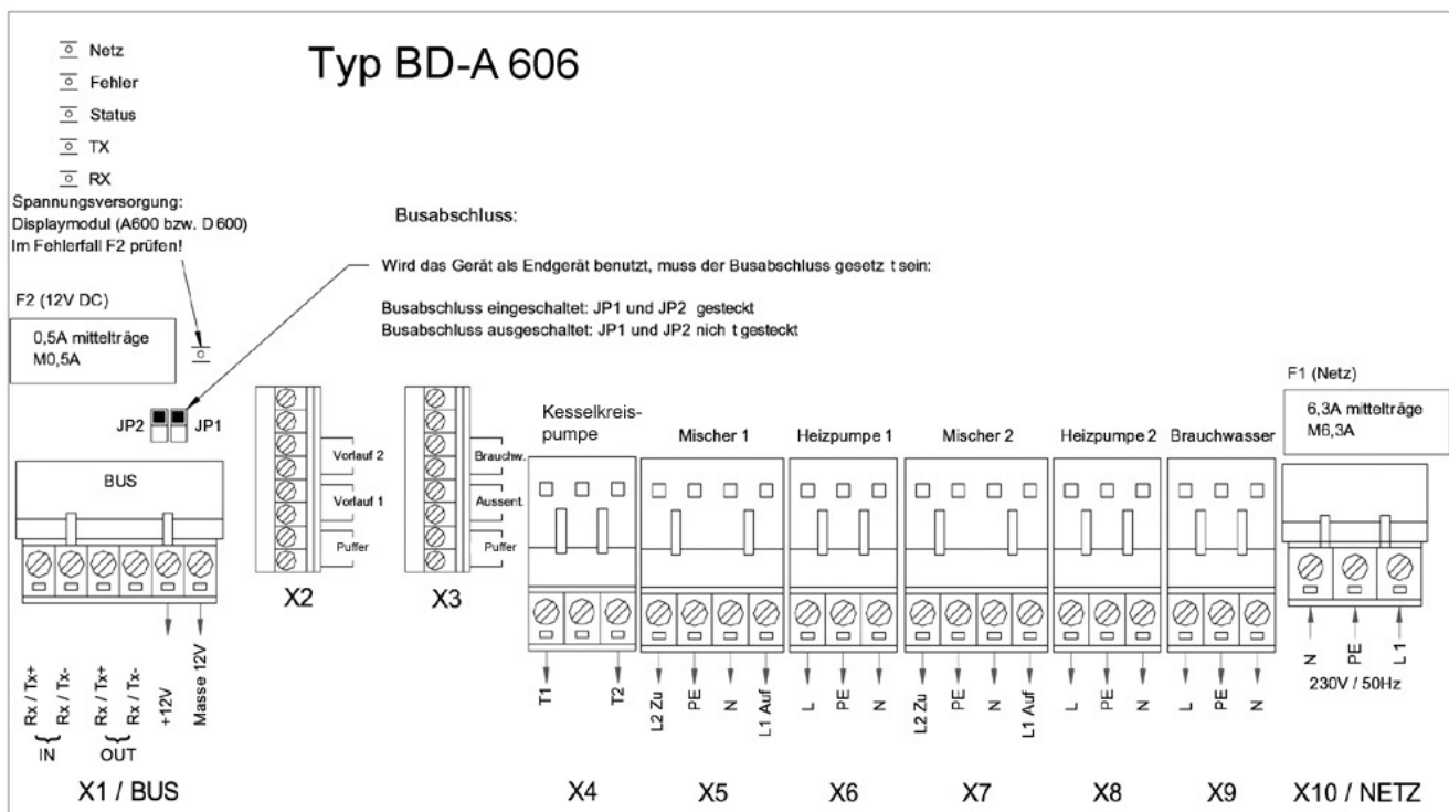
Abbildung 6: Anschlussplan
