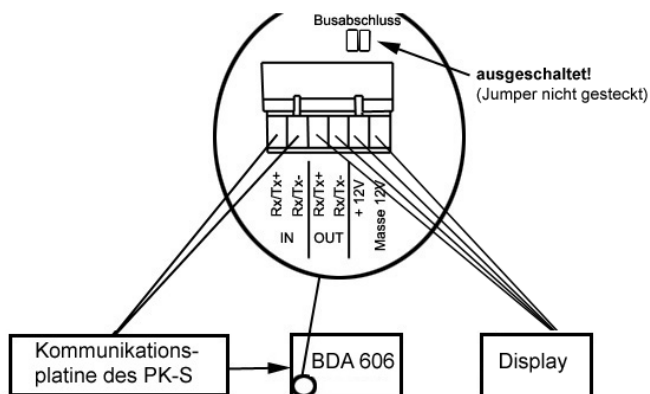
Abbildung 5: Kopplung Kommunikationsplatine, BD-A 606 und Display
